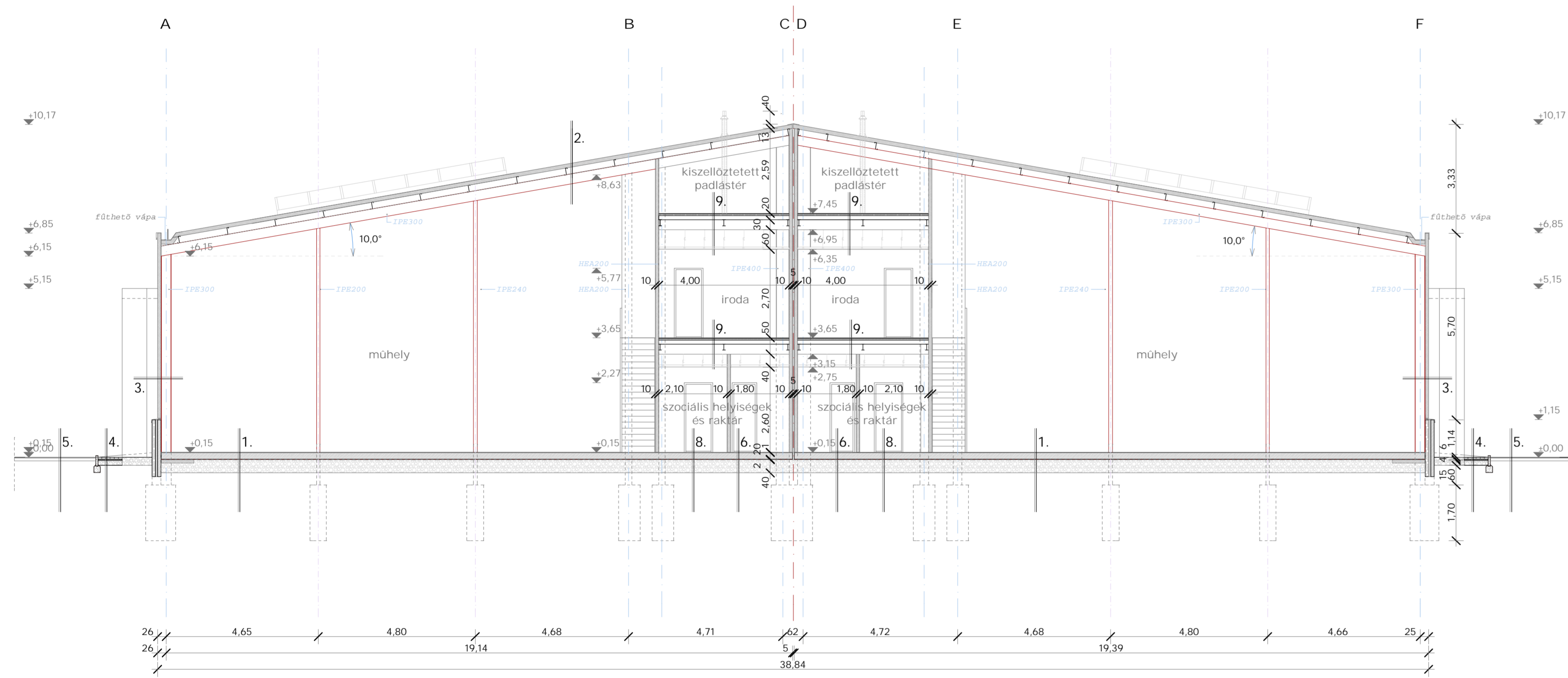
a-a metszet m=1:100
